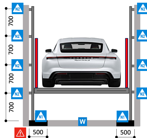
Querschnitt Liftschacht
