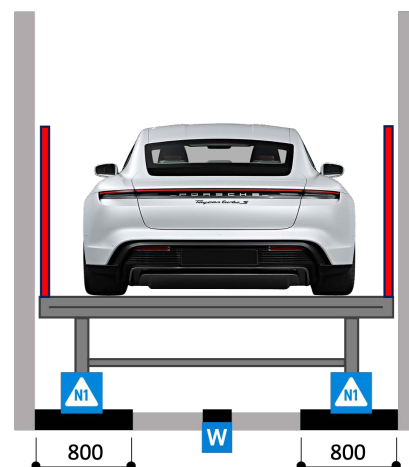
Querschnitt Liftschacht
